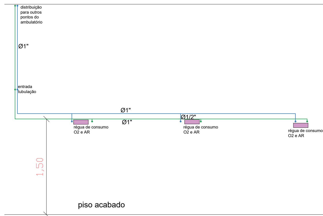
Vista esquemática Rede gases medicinal
