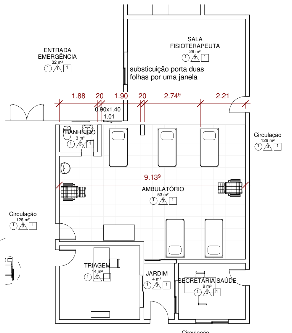
1 PLANTA BAIXA REFORMA 1 : 100
