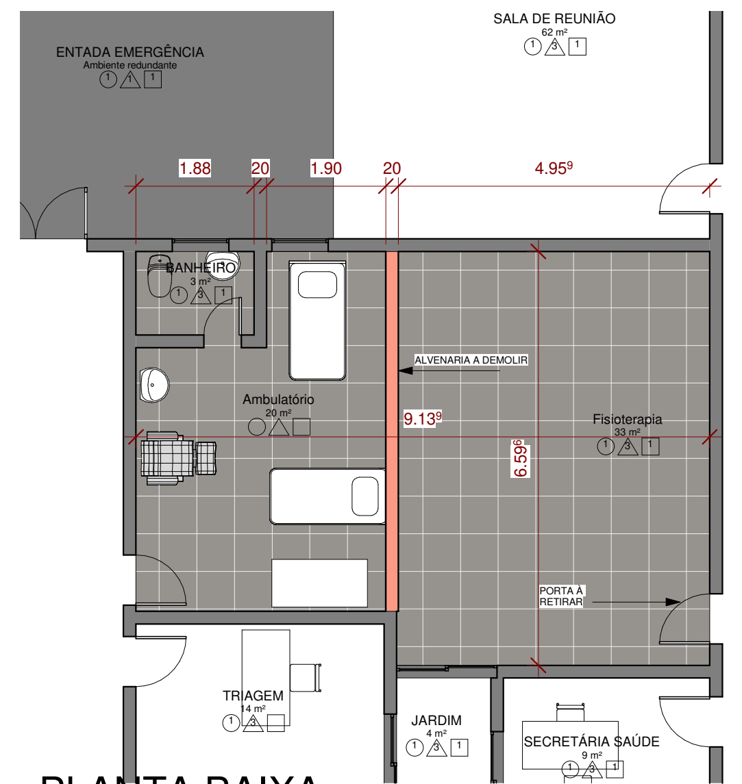
3 PLANTA BAIXA EXISTENTE 1 : 75
