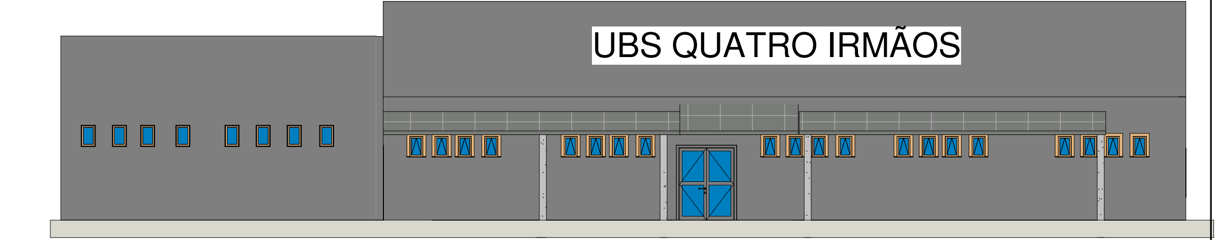
5 FACHADA FRONTAL 1 : 100
