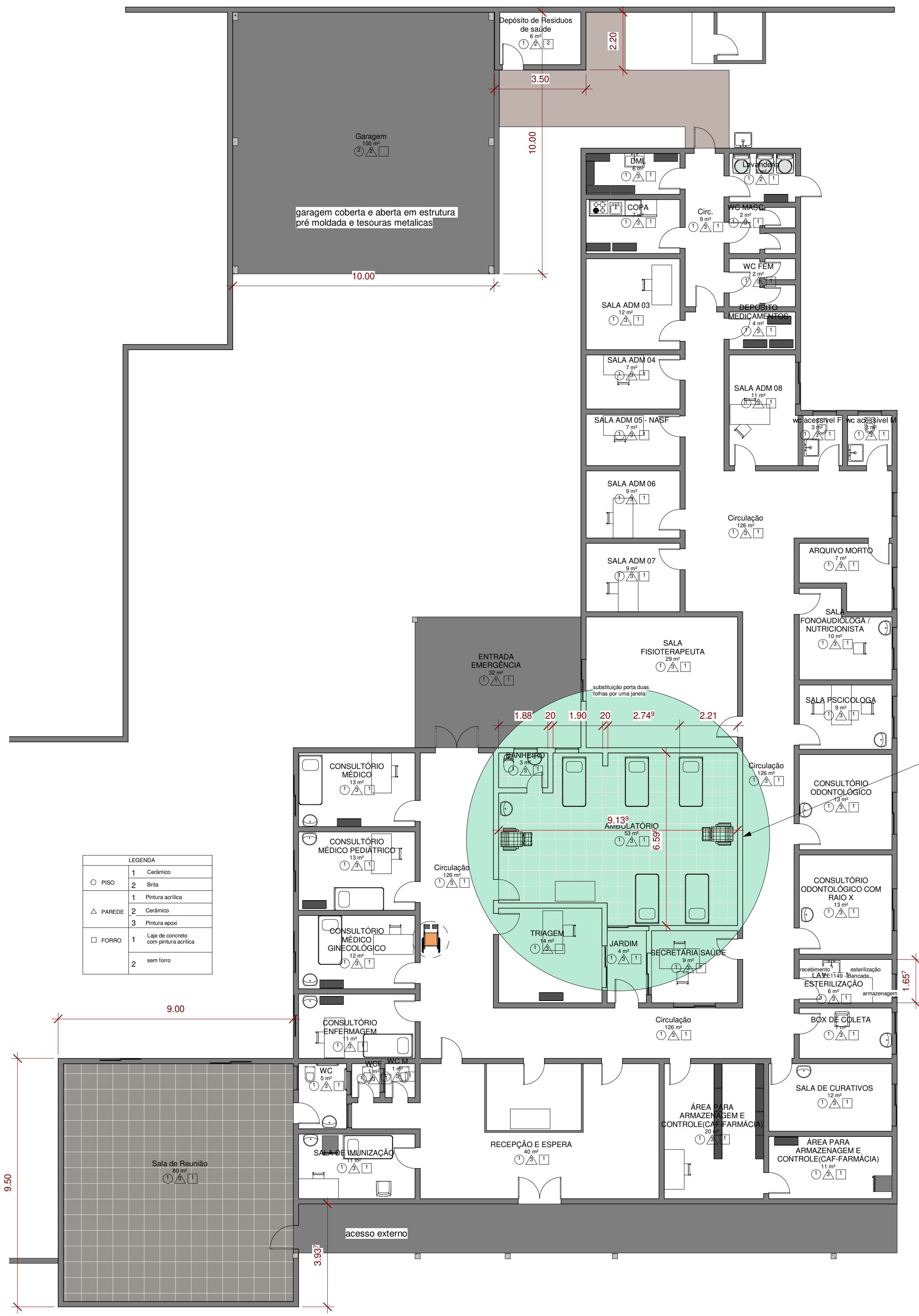
2 PLANTA BAIXA ARQUITETONICO 1 : 100
