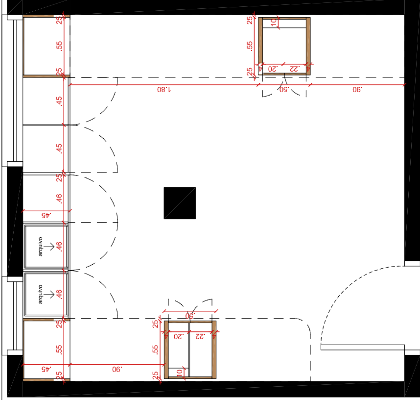
12 - PLANTA ESF - SEÇÃO 17 Esc: 1:25
