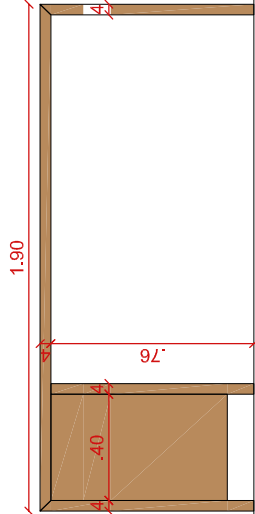
5- VISTA I3 Esc: 1:25
