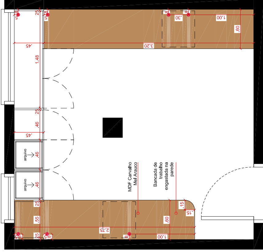
12 - PLANTA ESF - SEÇÃO 16 Esc: 1/25
