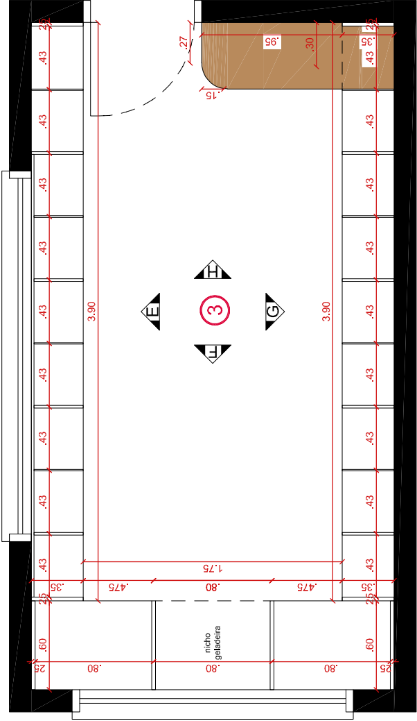
③- DEPÓSITO FARMÁCIA Esc: 1:25
