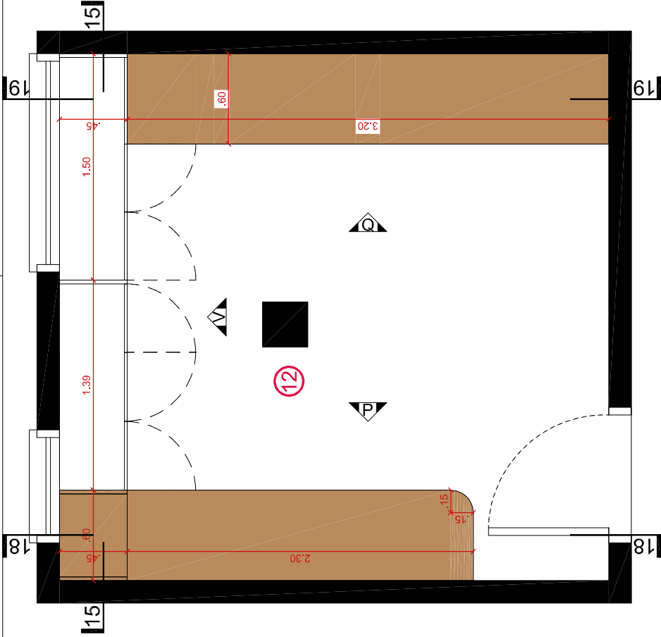
12 - PLANTA ESF Esc: 1/25
