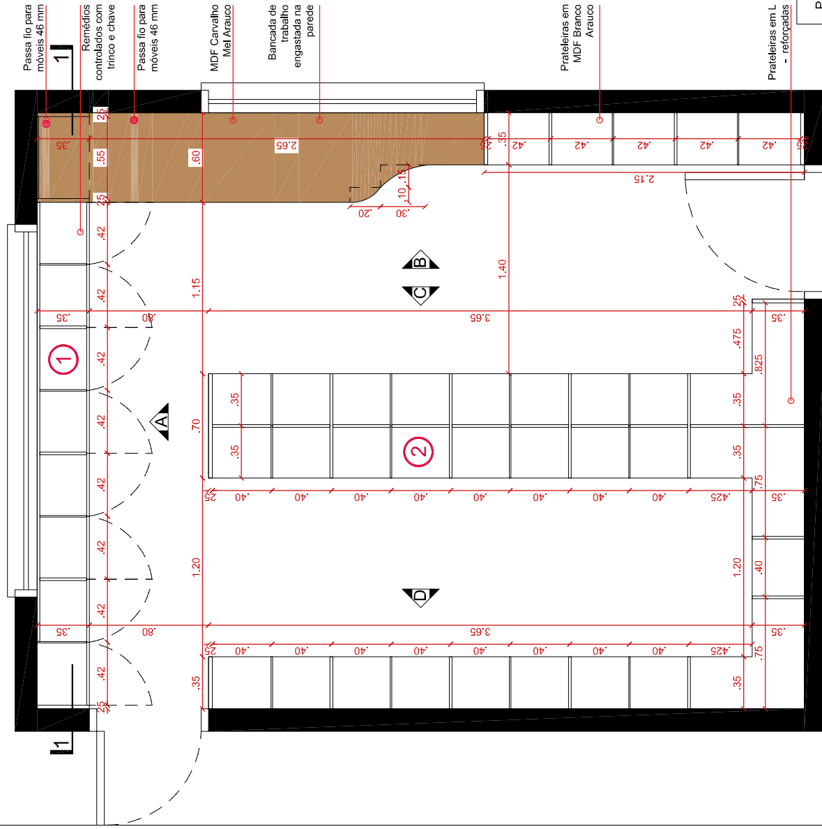
① ②-PLANTA FARMÁCIA Esc: 1:25
