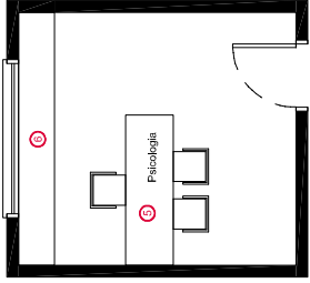
PLANTA ATENDIMENTO PSICO Esc: 1:75
