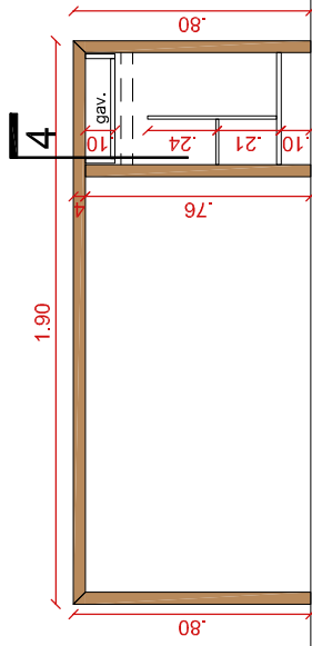
5- VISTA I1 SEM PORTAS Esc: 1:25
