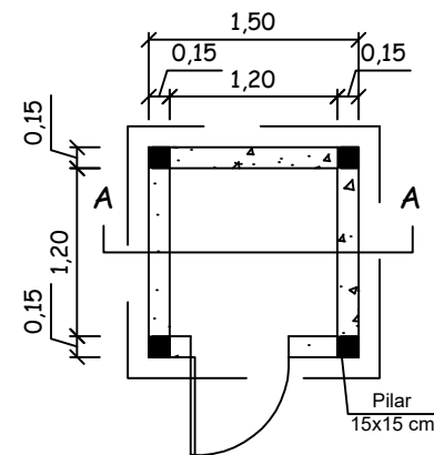
Planta Baixa Casa de Bombas
