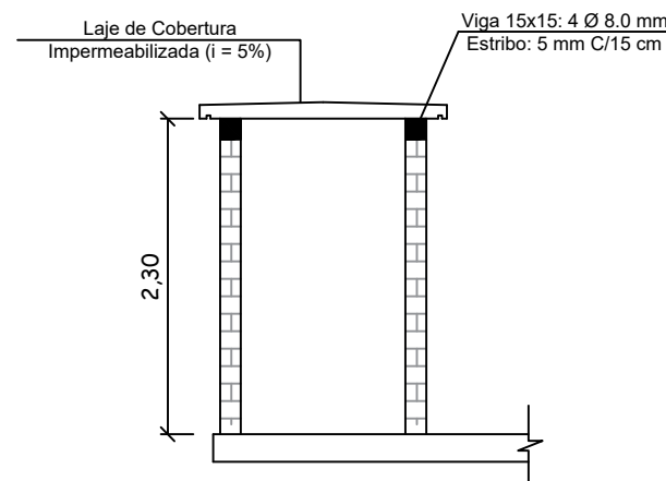
Corte A-A Casa de Bombas
