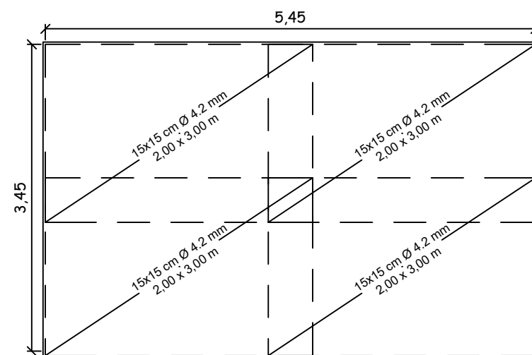
Disposição das Malhas Soldadas
