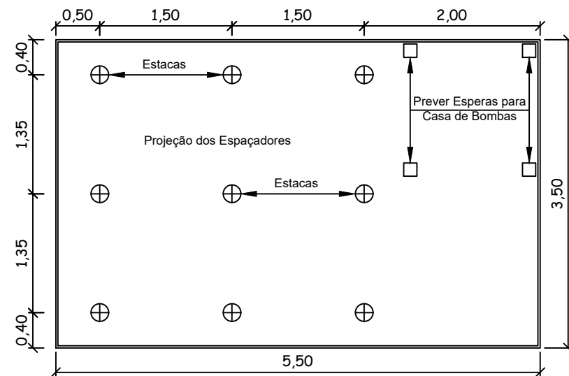
Planta Baixa Executiva
