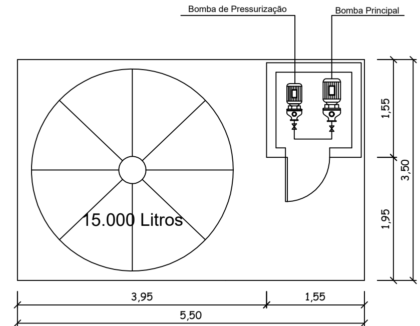
Planta Baixa
