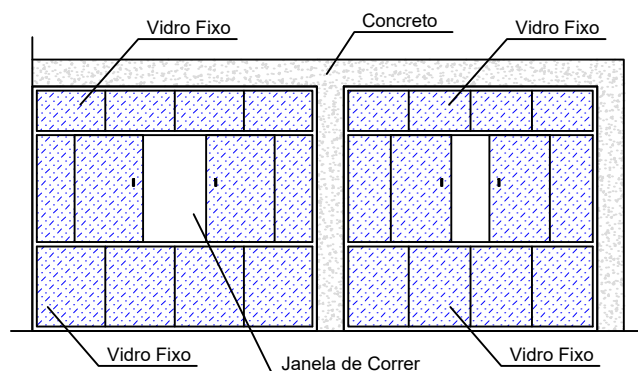
DETALHAMENTO - VISTA "A"
