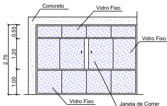
DETALHAMENTO - VISTA "B"
